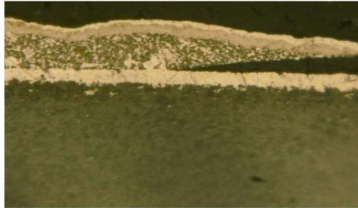
图 17 抗硫化产品研磨
