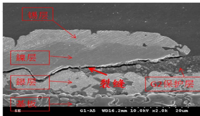
图 7 普通产品使用后出现裂缝
